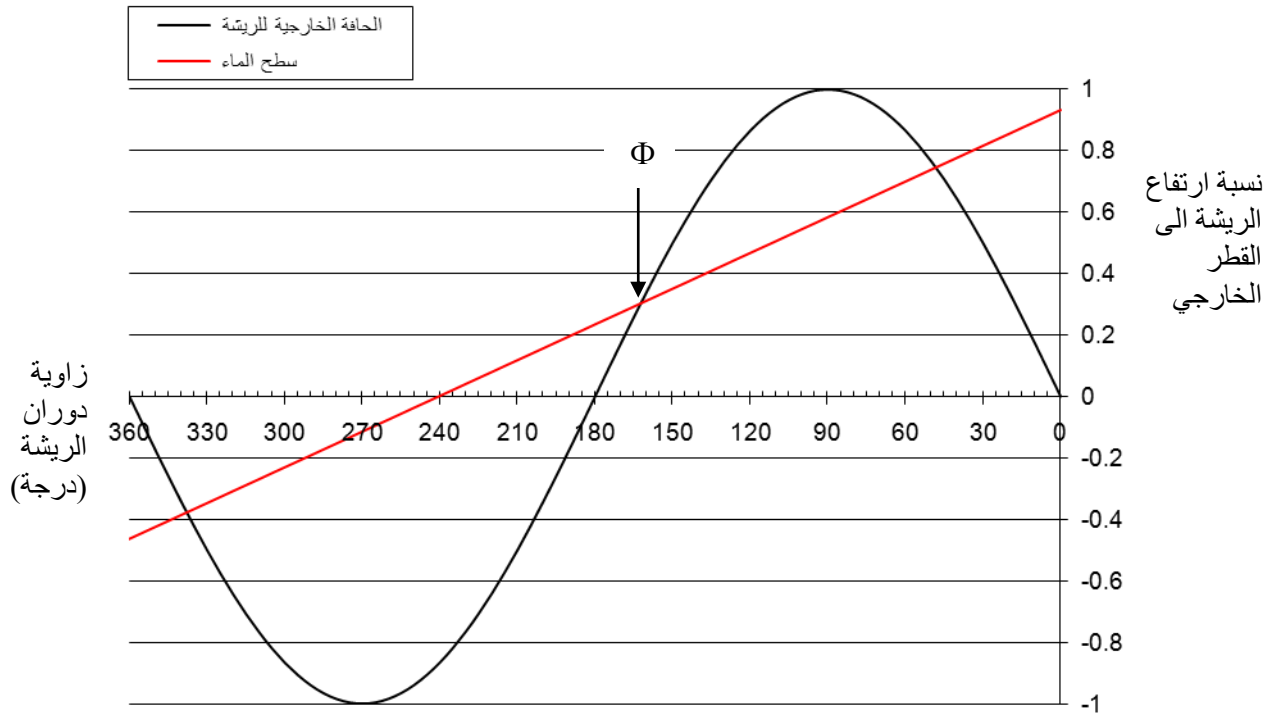
شكل رقم (9): شكل يبين الحافة الخارجية و سطح الماء للمضخة المقترحة.
