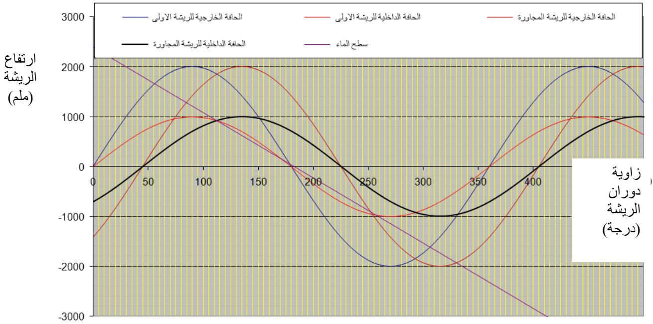
شكل رقم (6): شكل يبين ريشتين متجاورتين لمضخة فيتروفيوس و مستوى سطح الماء.
