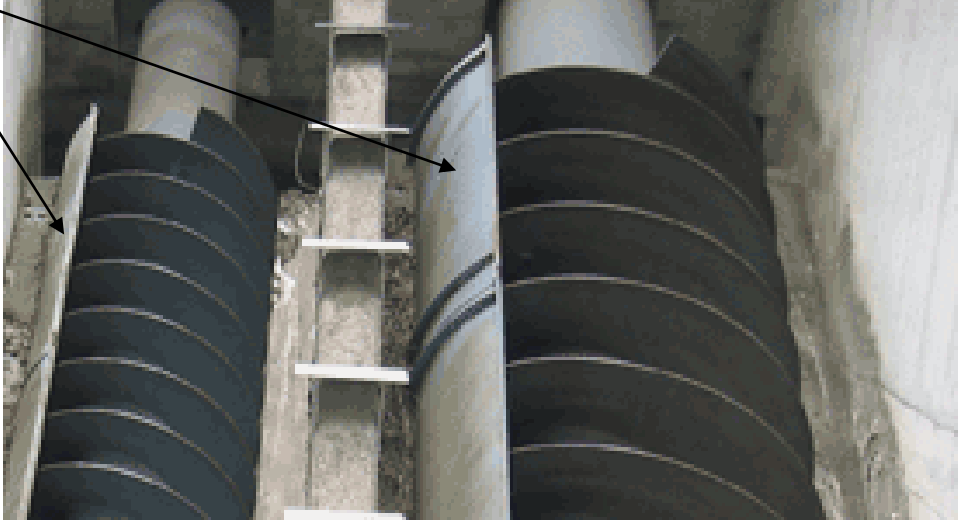
صورة (1): صورة توضح استخدام صفيحة التوجيه
