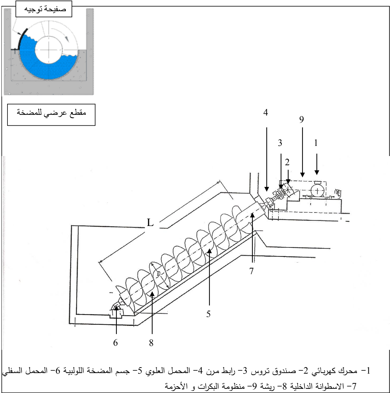
شكل رقم (1): شكل تخطيطي يوضح أجزاء المضخة اللولبية
