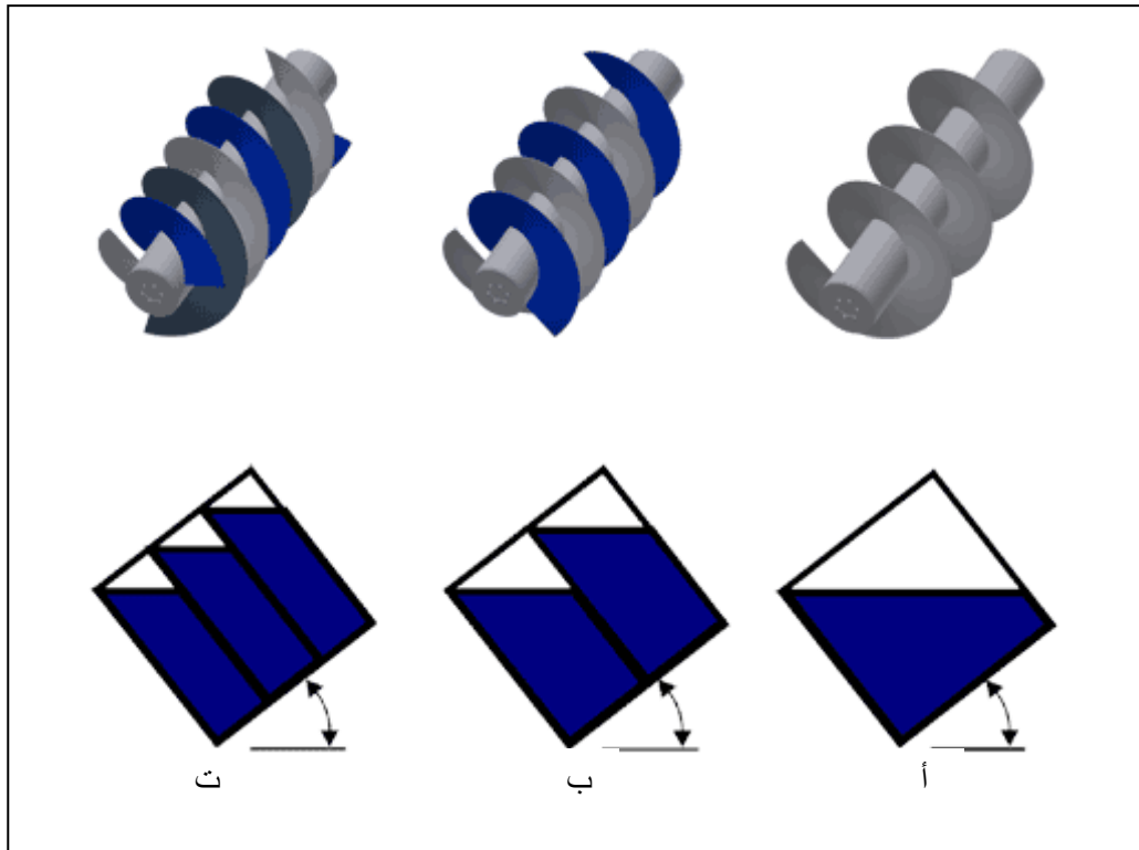
شكل رقم (3): شكل تخطيطي لثلاث مضخات يبين تأثير عدد الريش على تصريف المضخة ( المساحة الغامقة تمثل الجيوب المائية) 6
