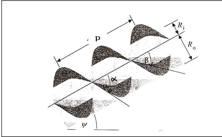
شكل رقم (5): شكل تخطيطي لقطعة من مضخة لولبية ذات ريشتين 8
