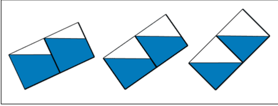
شكل رقم (4): شكل تخطيطي يوضح تأثير زاوية ميلان المضخة عن الأفق على تصريفها (المنطقة الغامقة تمثل الجيوب المائية) 6
