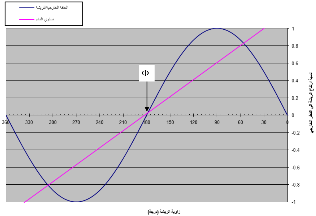
شكل رقم (7): شكل يبين تقاطع سطح الماء مع الحافة الخارجية للريشة الأولى لمضخة فيتروفيوس.
