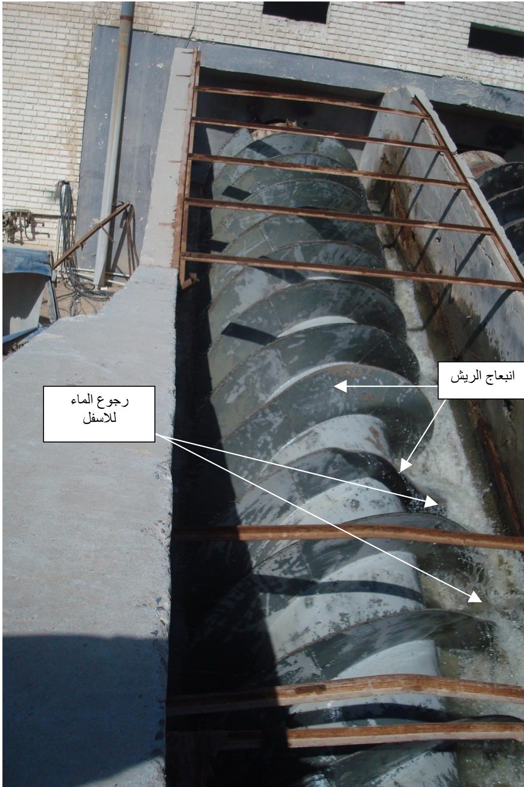
صورة (3): صورة قريبة للمضخة
