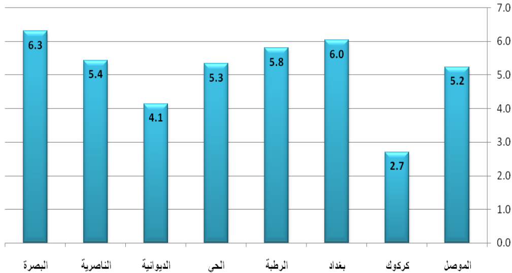
شكل (٢) يبين التوزيع المكاني لنسبة التغطية أثناء حدوث العواصف الرعدية غير الممطرة للمدة من ١٩٩١ - ٢٠٠٢
