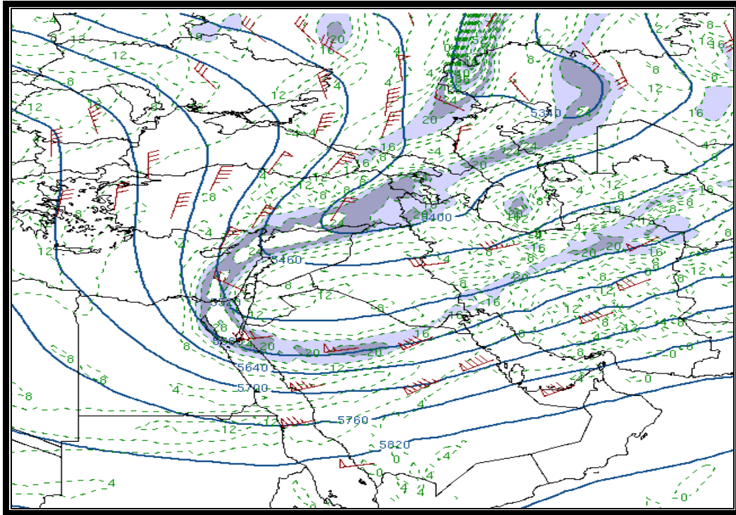
شكل (٨) أخدود (Trough) سيبيري عميق ضمن مستوى (٥٠٠) مليبار يغطي منطقة الدراسة (الساعة ١٢ ليلا) يوم ٢٦/١/٢٠١٦
