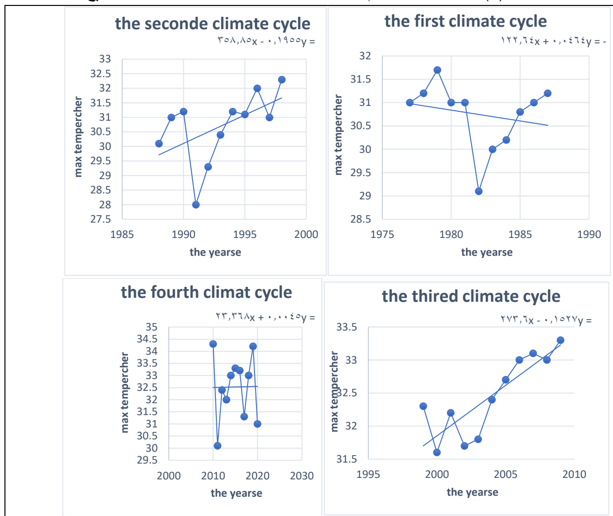
شكل (٣) معامل الاتجاه العام لدرجات الحرارة الصغرى للدورات المناخية الاربع
